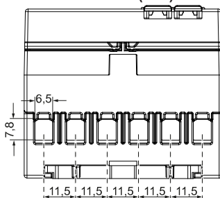
Untersicht (mm)
